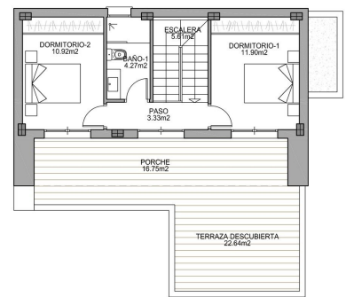
PLANTA PRIMERA
